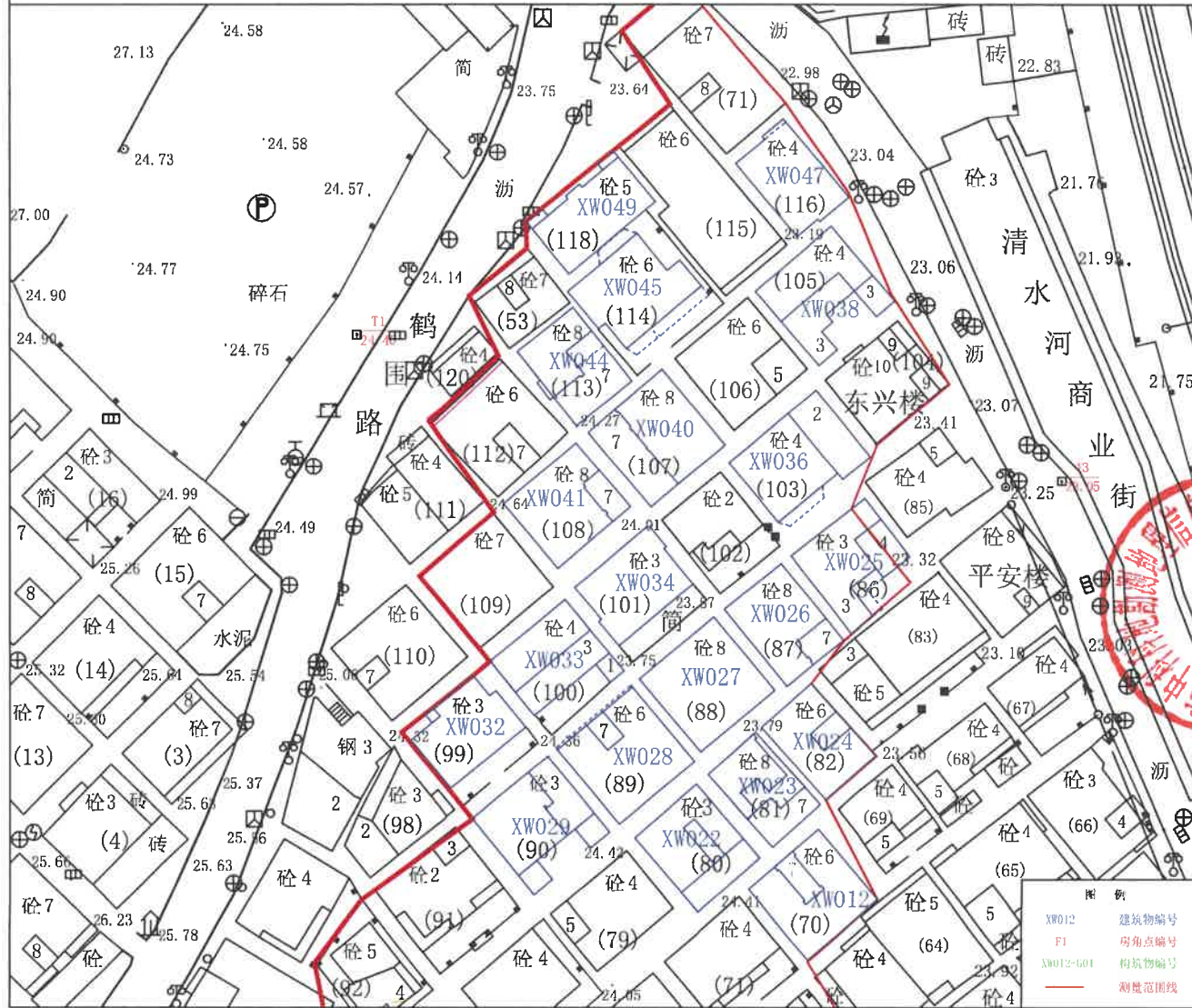
深圳地铁17号线一期工程罗湖北站至德兴站区间施工涉及房屋建筑物信息图
