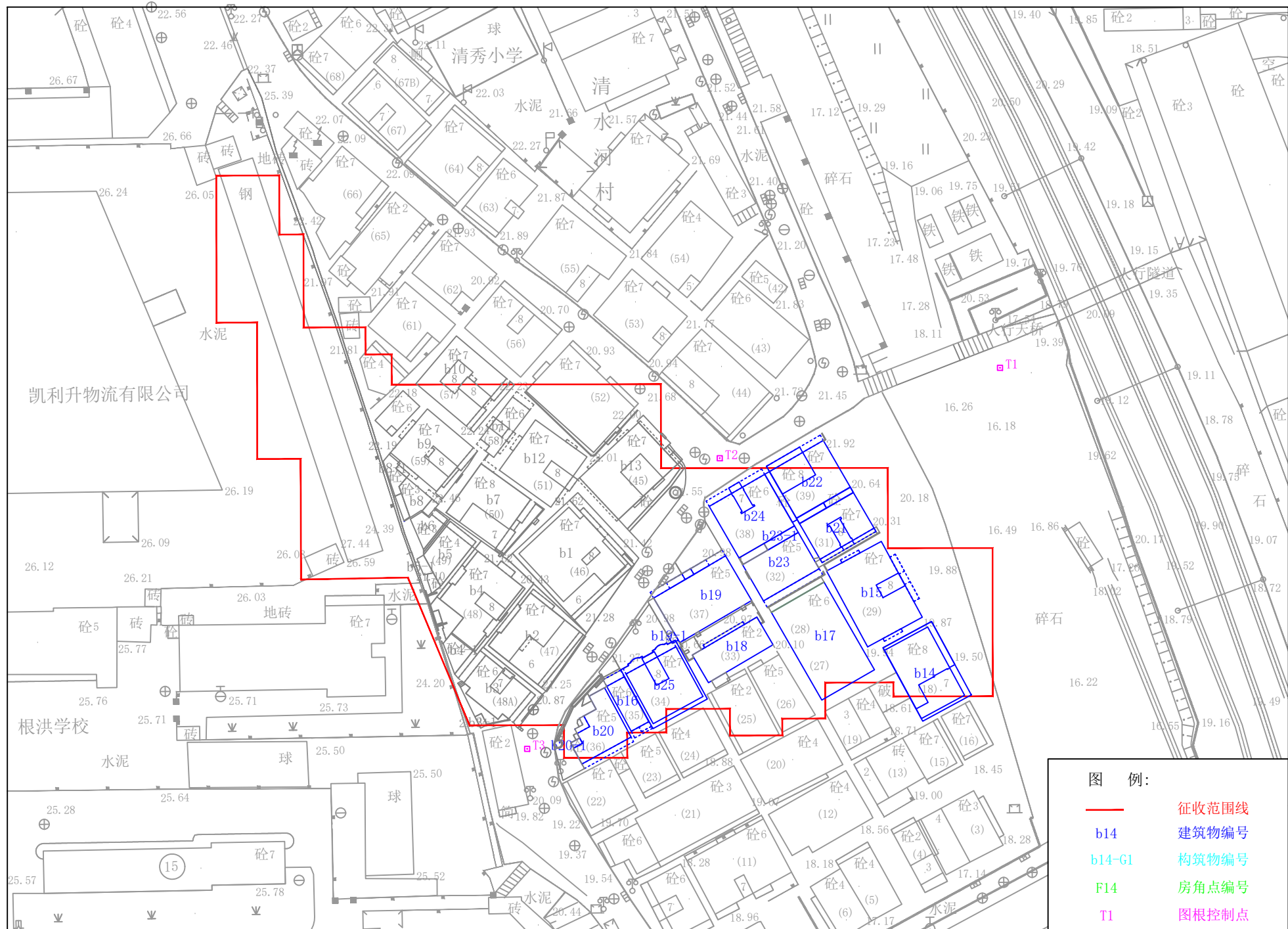
深圳至深汕合作区铁路项目（罗湖北站）涉及清水河村建筑物信息图
