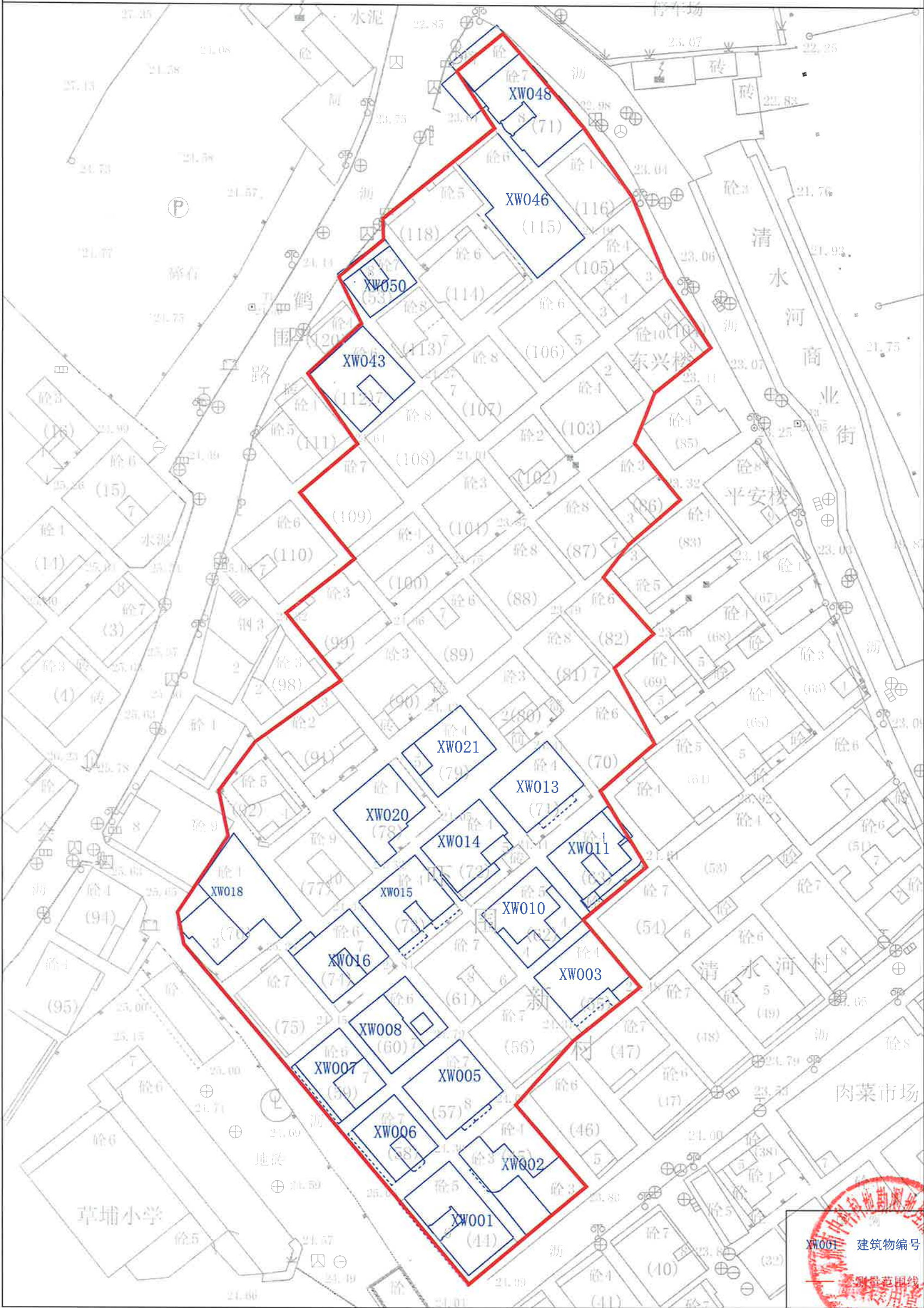
深圳地铁17号线一期工程罗湖北站至德兴站区间施工涉及房屋建筑物信息图
