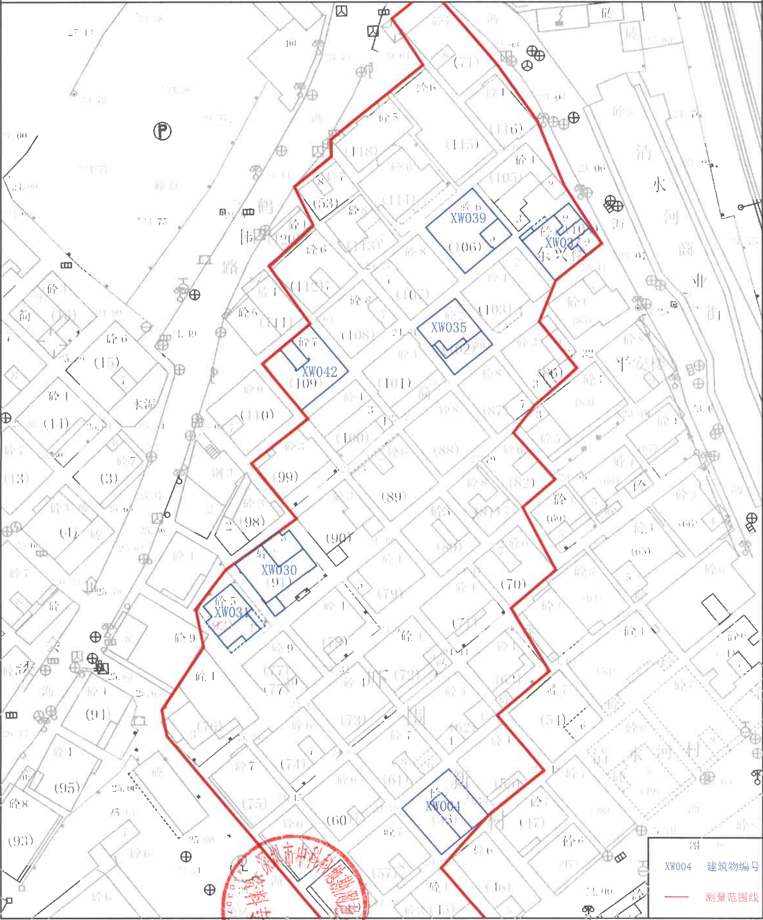
深圳地铁17号线一期工程罗湖北站至德兴站区间施工涉及房屋建筑物信息图
