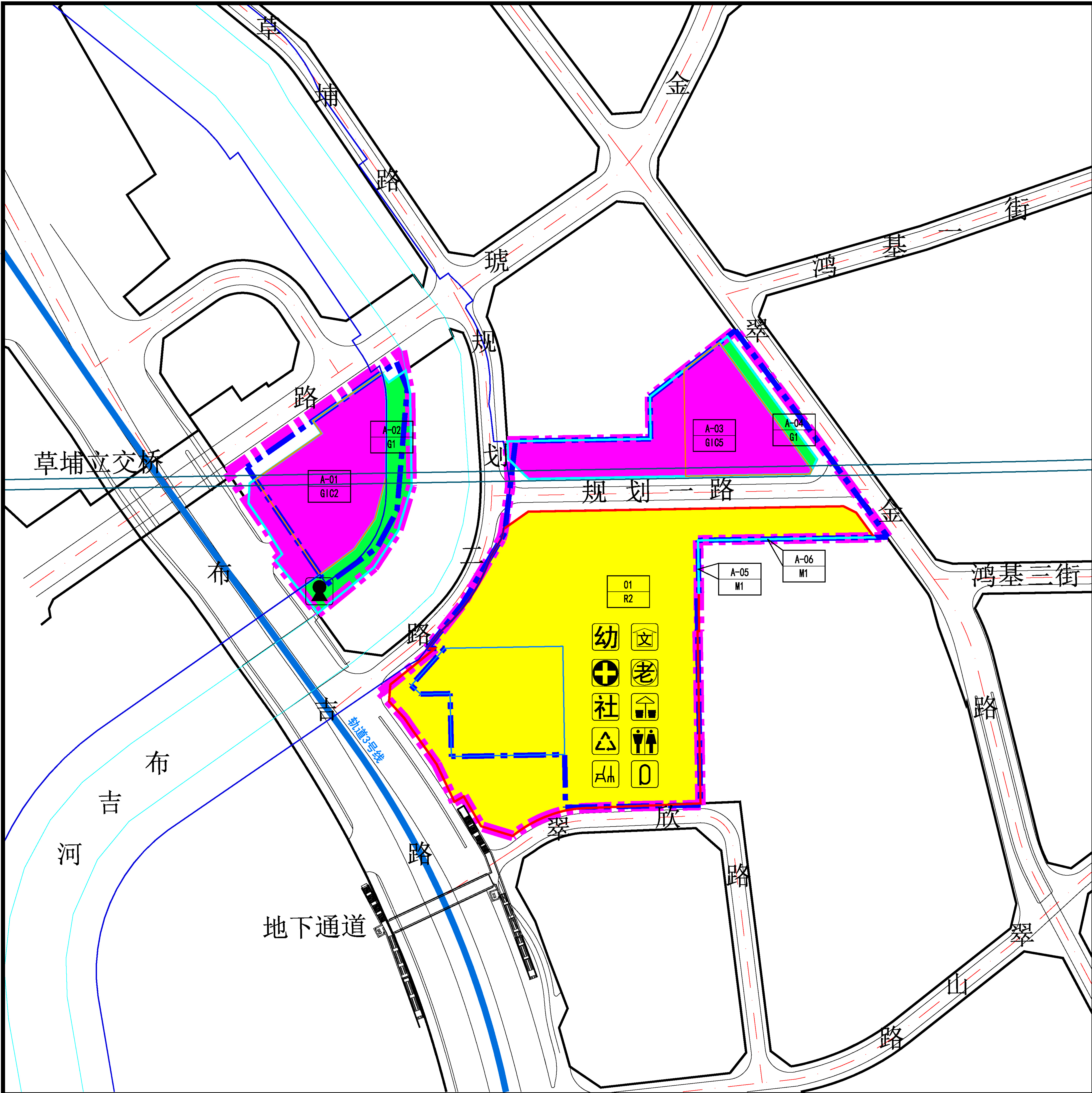
地块划分与指标控制图
